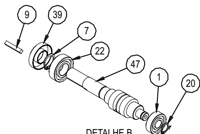
DETALHE B ESCALA 2 : 5
