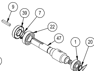
DETALHE B ESCALA 2 : 5
